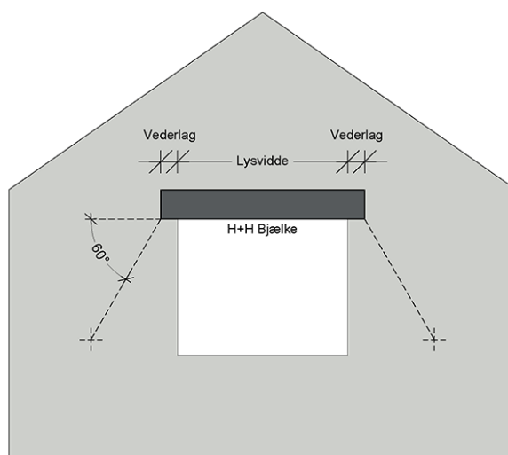
Figur 2. Bjælke i gavl.
