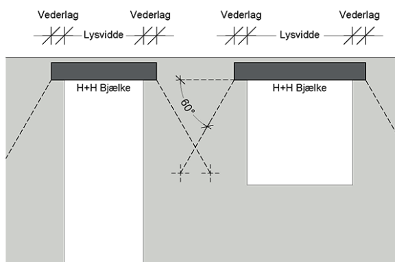
Figur 3. Bjælker i facade.
