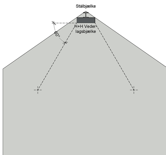
Figur 6. Vederlagsbjælke under stålbjælke i gavl.
