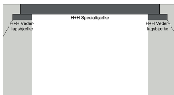
Figur 4. Specialbjælke og vederlagsbjælker i facade.
