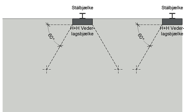
Figur 5. Vederlagsbjælke under stålbjælke i facade/skillevæg.
