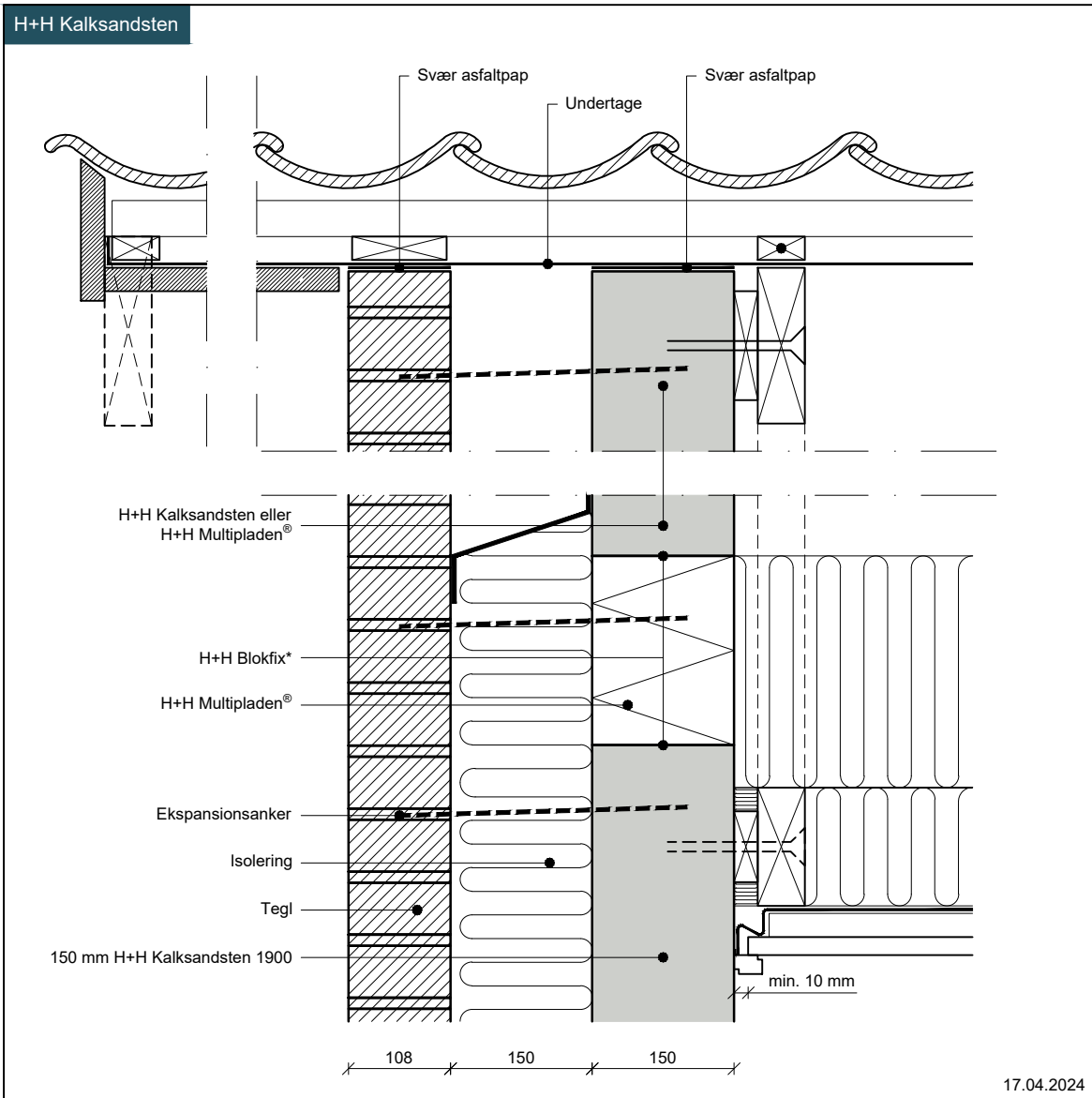
TEGNINGSNUMMER: GA500-KS
