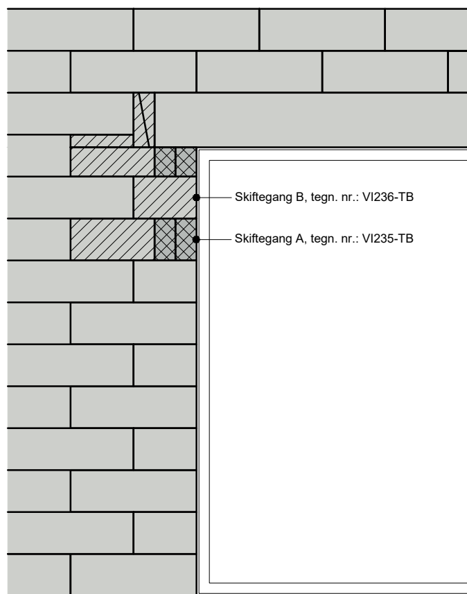
Opstalt, indvendig, 1:25
