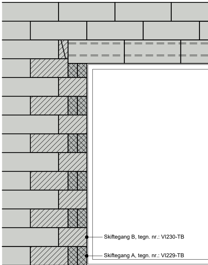
Opstalt, indvendig, 1:25
